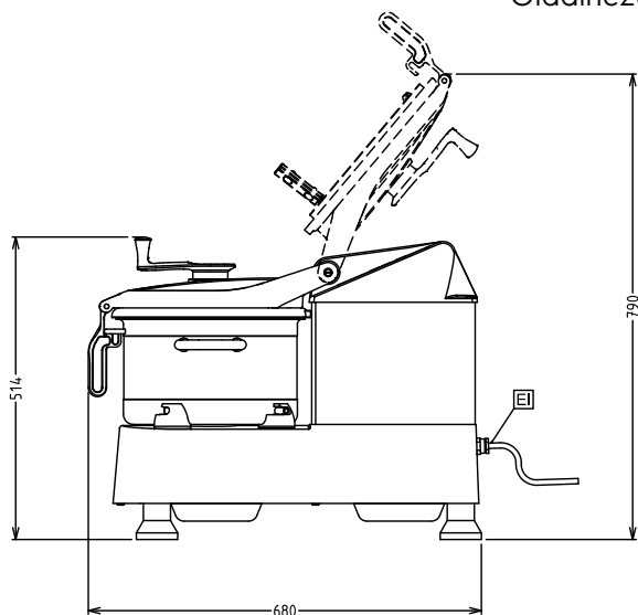
Oldalnézet
